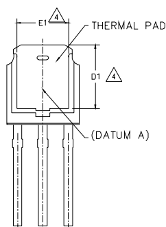
VIEW A-A
