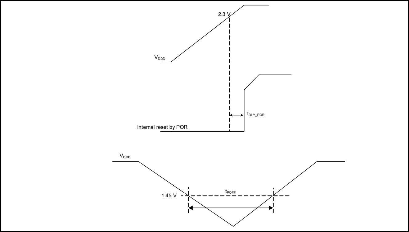
Figure 26-15 POR specifications
