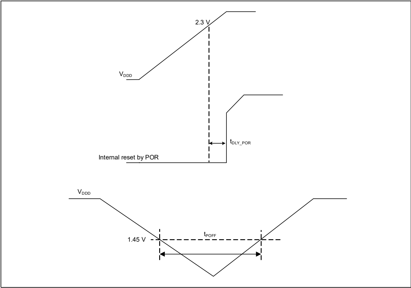
Figure 26-15 POR specifications
