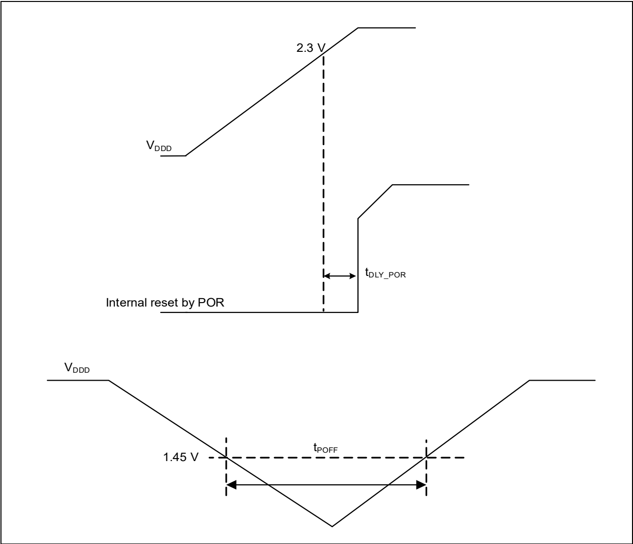
Figure 27-15 POR specifications
