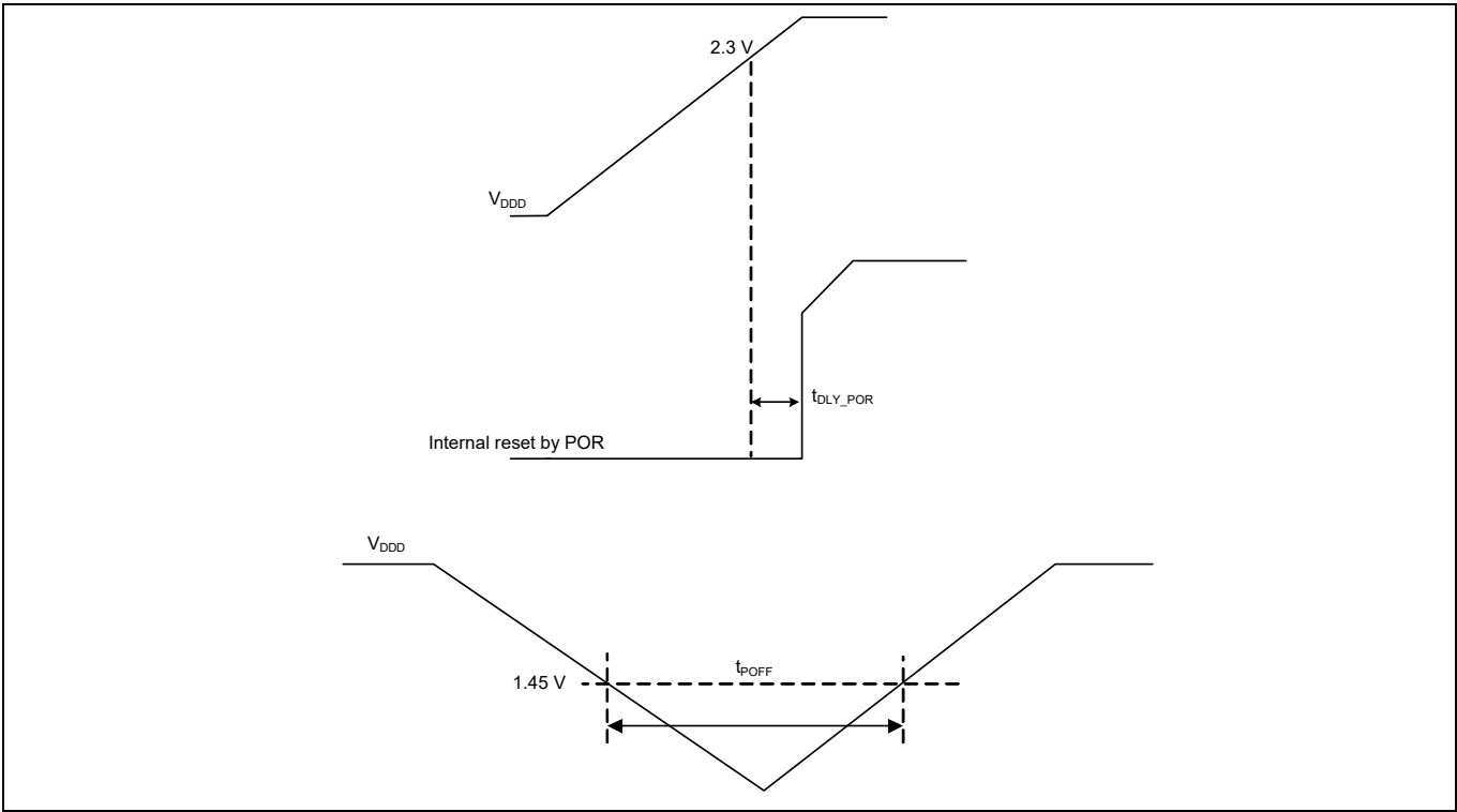
Figure 27-15 POR specifications
