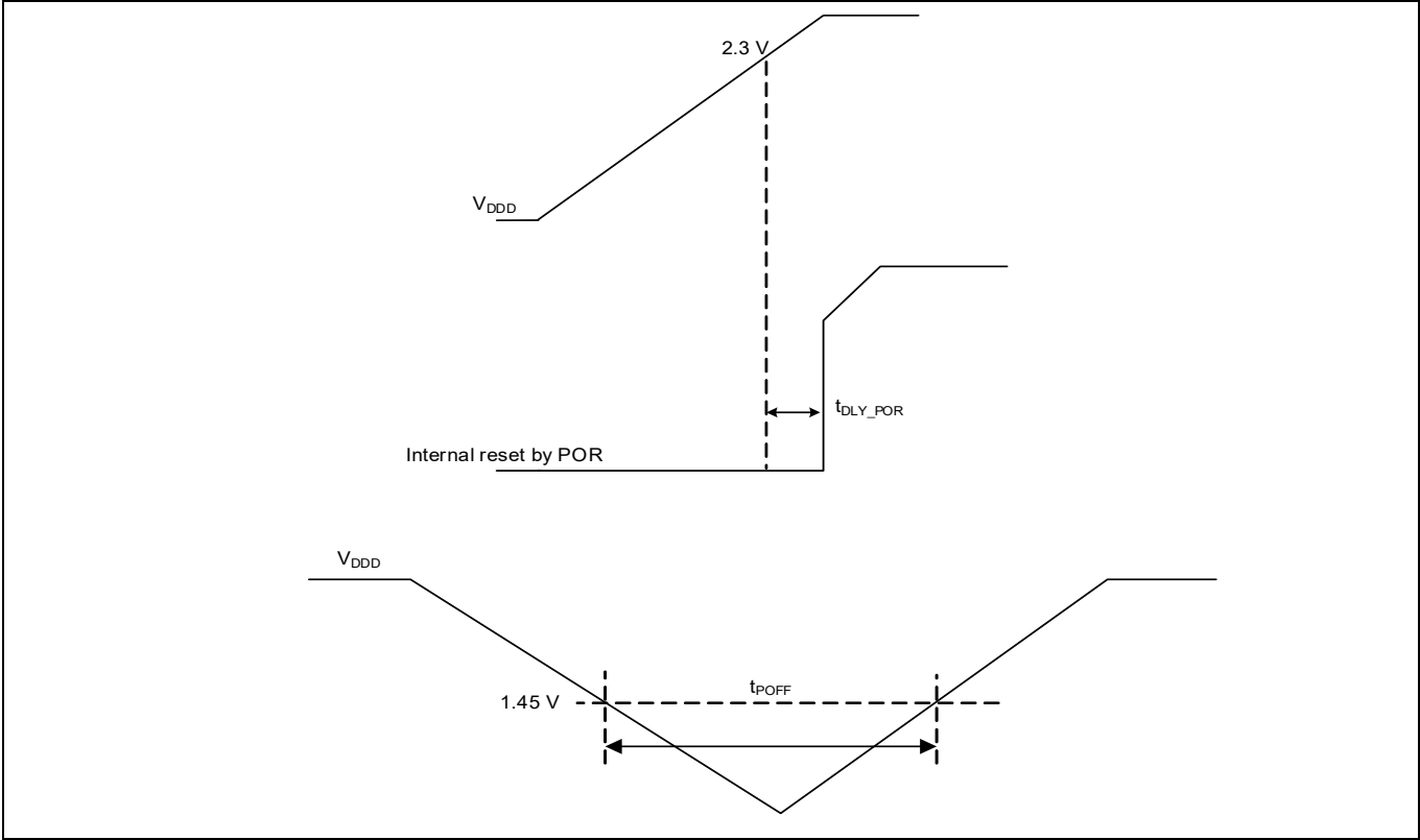
Figure 27-16 POR specifications
