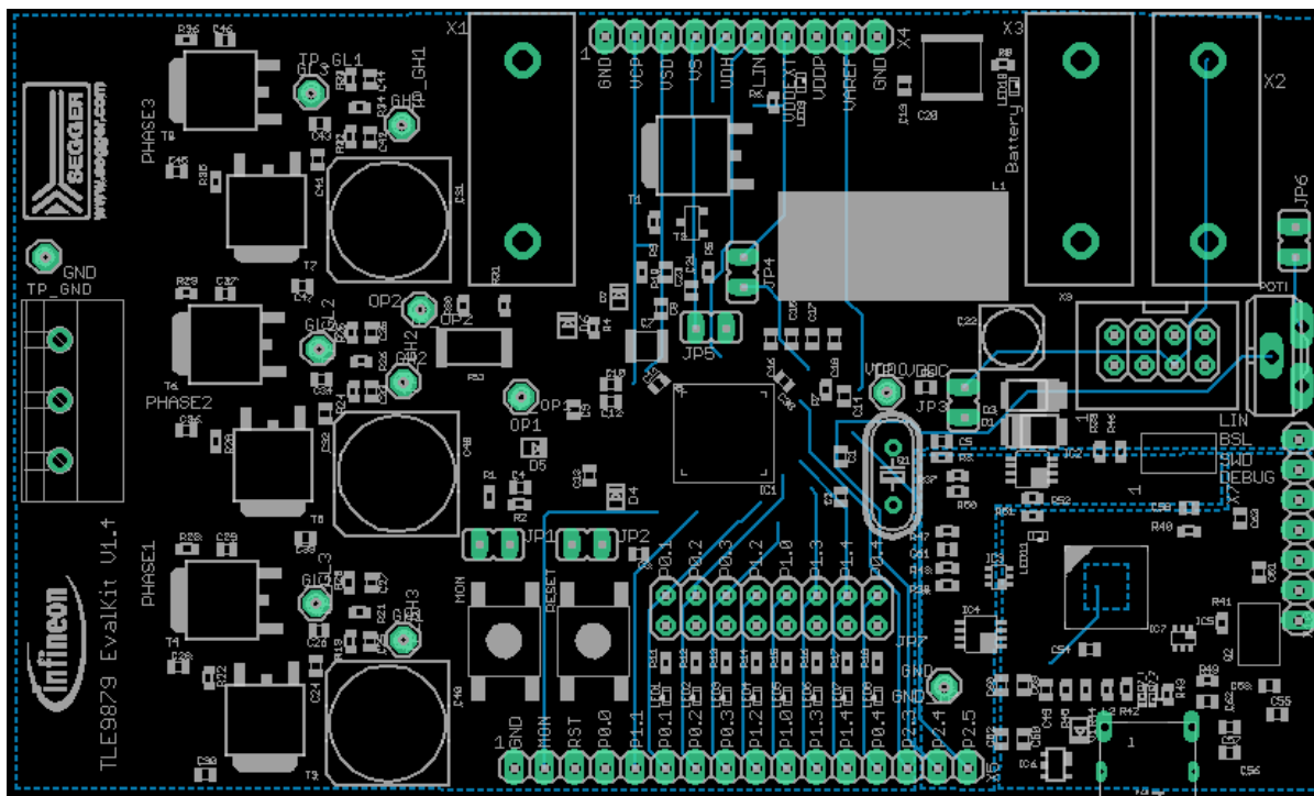
Bottom Layer
