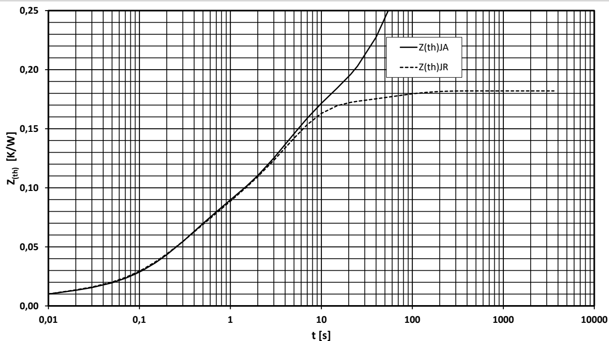
Transienter Wärmewiderstand je Zweig / Transient thermal impedance per arm
