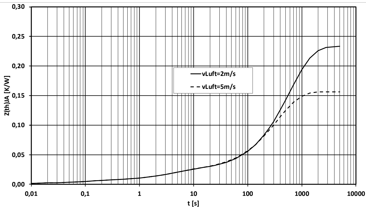
Transienter Wärmewiderstand je Zweig / Transient thermal impedance per arm Z_{thJA} = f(t)
