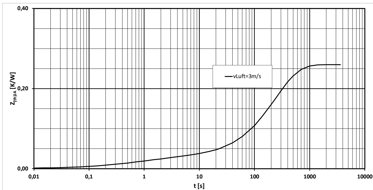
Transienter Wärmewiderstand je Zweig / Transient thermal impedance per arm Z_{thJA} = f(t)
