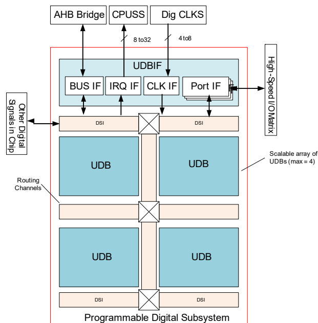
図 5. UDB アレイ
