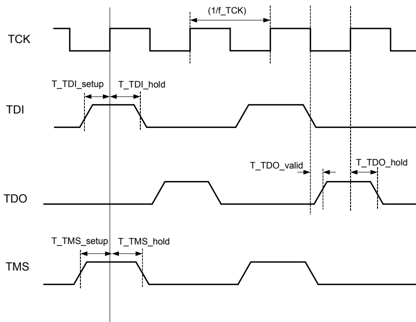
图 11-68. JTAG 接口时序
