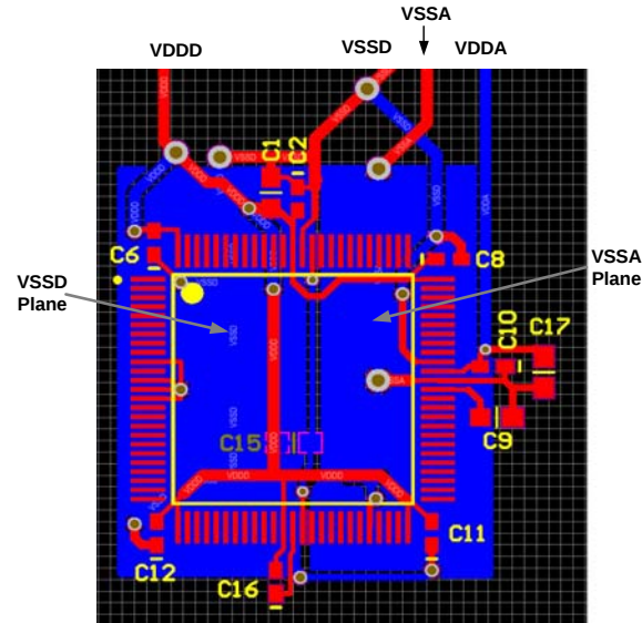
图 2-8. 100-TQFP 器件获得最佳模拟性能的 PCB 布局示例
