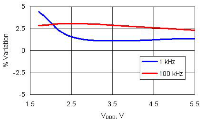
图 11-74. ILO 频率变化与 V_{DD}
