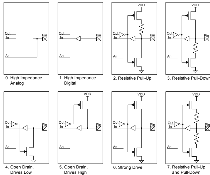
图 6-12. 驱动模式
