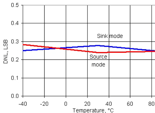
图 11-39. IDAC DNL 与温度，范围 = 255 \mu A，高速模式
