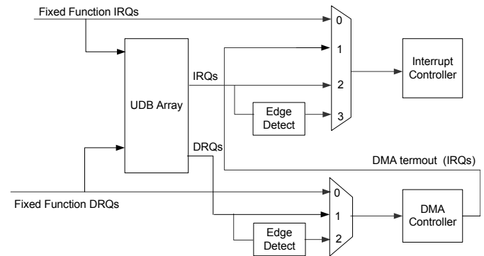
图 7-10. IDMUX 中的中断和 DMA 处理
