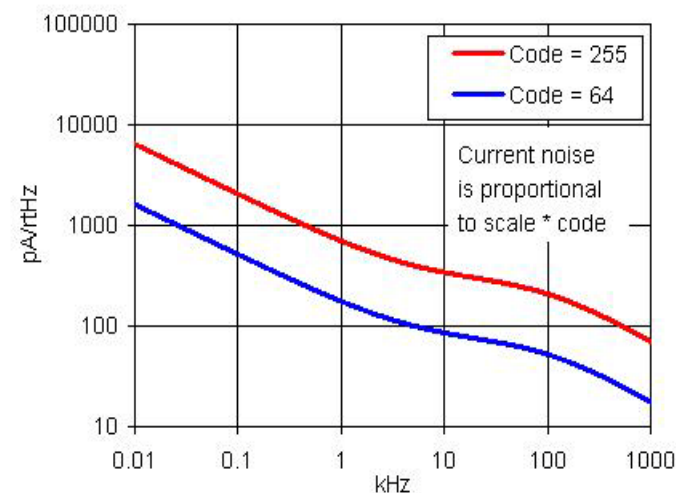
图 11-47. IDAC 当前噪声, 255 \mu A 模式, 拉电流模式, 高速模式, V_{DDA} = 5 V
