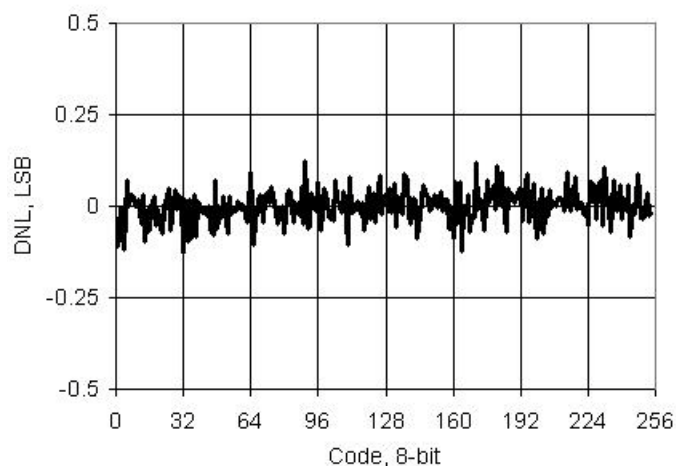
图 11-37. IDAC DNL 与输入代码，范围 = 255 \mu A，灌电流模式
