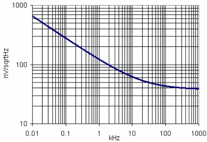
图 11-30. 运算放大器噪声与频率, 功耗模式 = 高, V_{DDA} = 5\text{ V}
