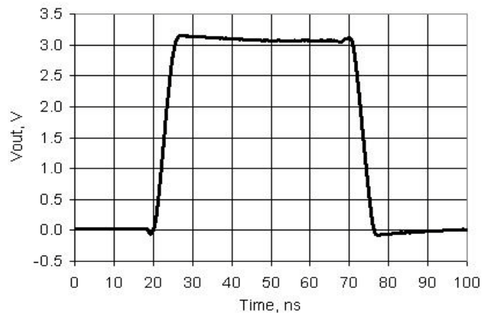
图 11-24. USBIO 输出上升和下降时间, GPIO 模式, V_{DD} = 3.3\text{ V} , 25 pF 负载
