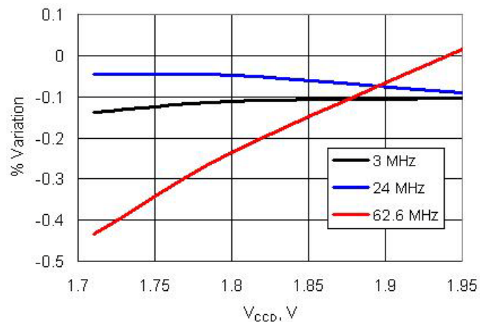
图 11-72. IMO 频率变化与 V_{CC}
