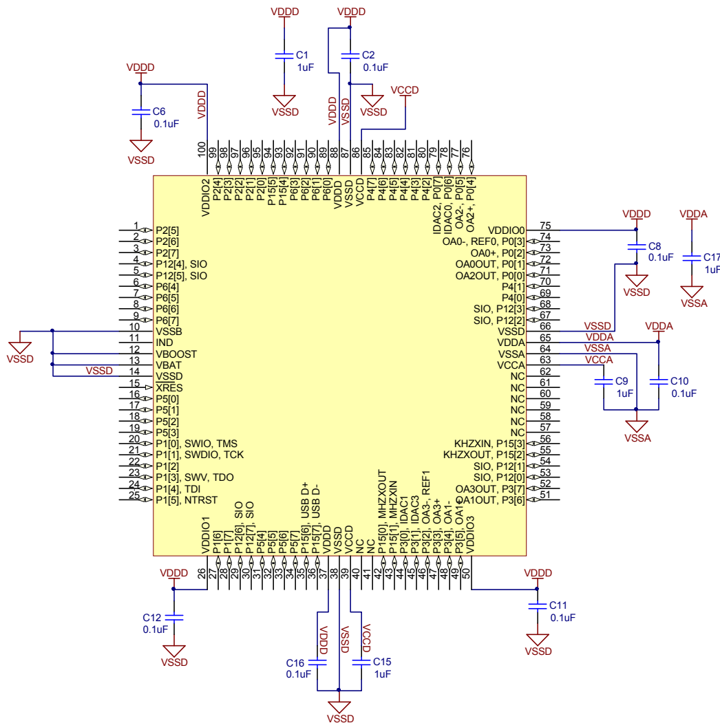
图 2-7. 100-TOFP 器件的原理图示例 (包含供电连接)
