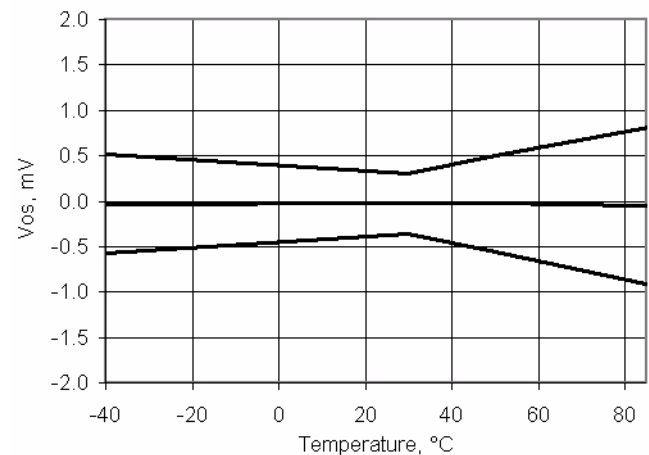
图 11-26. 运算放大器偏移与温, V_{\text{DDA}} = 5\text{ V}
