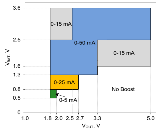
图 11-9. 与 V_{\text{BAT}} 和 V_{\text{OUT}} 相比的 I_{\text{OUT}} 范围
