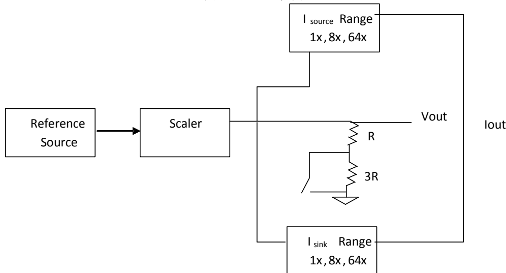
图 8-11. DAC 框图
