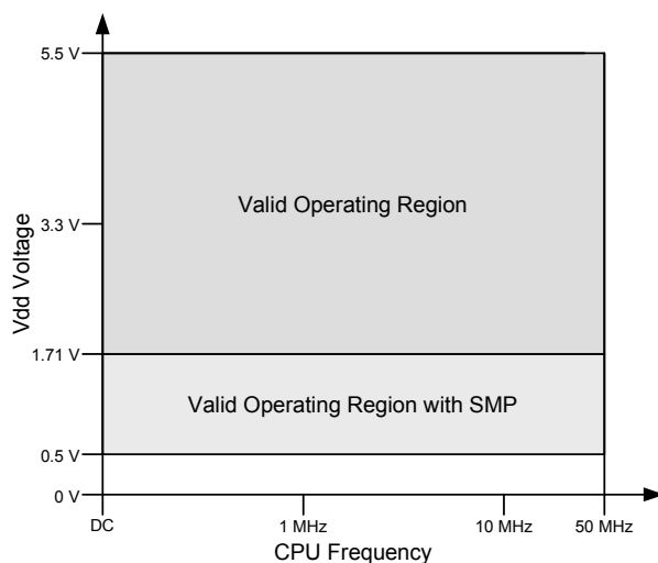
图 11-4. F_{CPU} 与 V_{DD}
