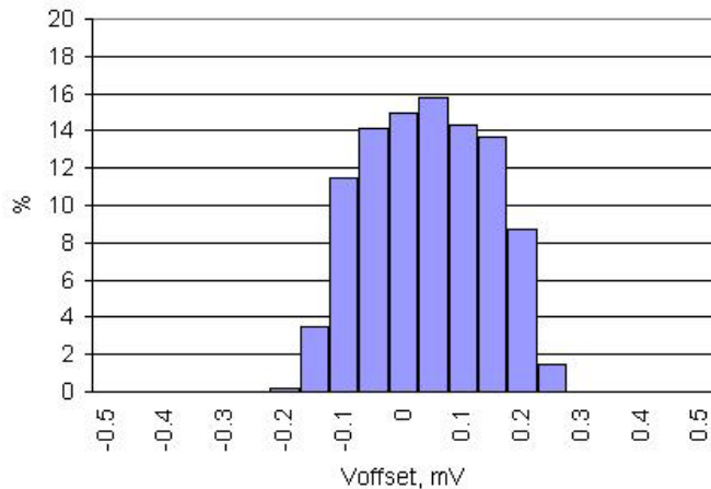
图 11-25. 运算放大器偏移柱状图, 3388 个采样 / 847 个器件, 25^{\circ}\text{C} , V_{\text{DDA}} = 5\text{ V}
