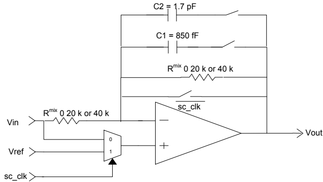
图 8-12. 混频器配置
