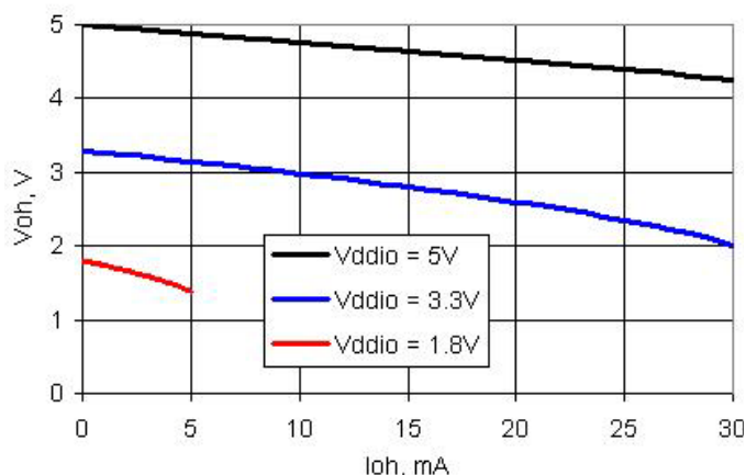
图 11-17. SIO 输出高电平和电流，非稳压模式
