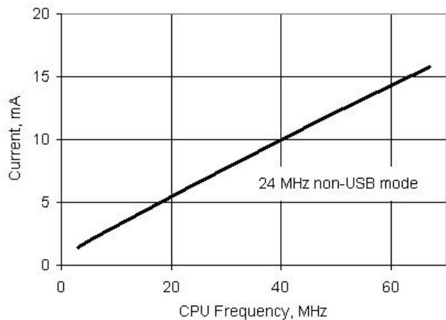
图 11-1. 活动模式电流与 F_{CPU} , V_{DD} = 3.3\text{ V} , 温度 = 25\text{ }^{\circ}\text{C}
