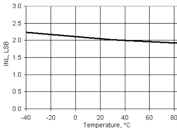
图 11-54. VDAC 工作电流与温度, 1 V 模式, 低速模式
