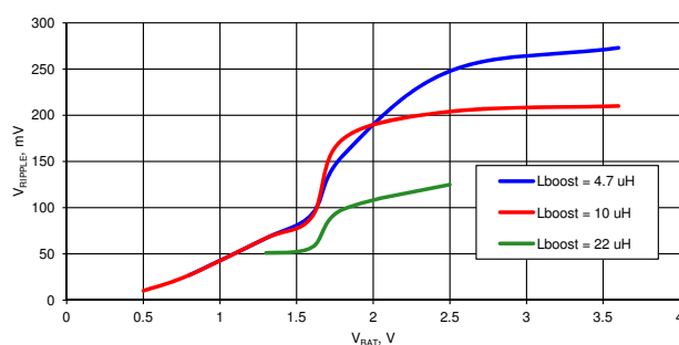
图 11-14. V_{RIPPLE} 与 V_{BAT} [37]
