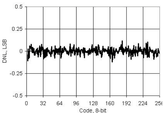
图 11-49. VDAC DNL 与输入代码，1 V 模式
