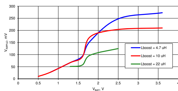
图 11-14. V_{RIPPLE} 与 V_{BAT} [34]
