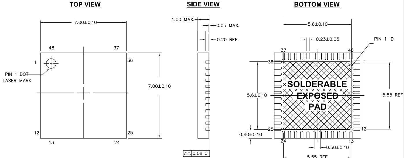
图 13-2. 48-QFN 封装外形
