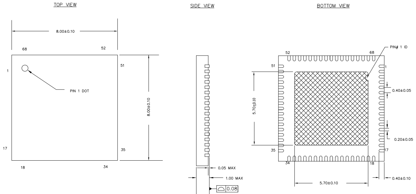
图 13-3. 间距为 0.4 毫米的 68-QFN 8×8 封装外形 (Sawn 版本)
