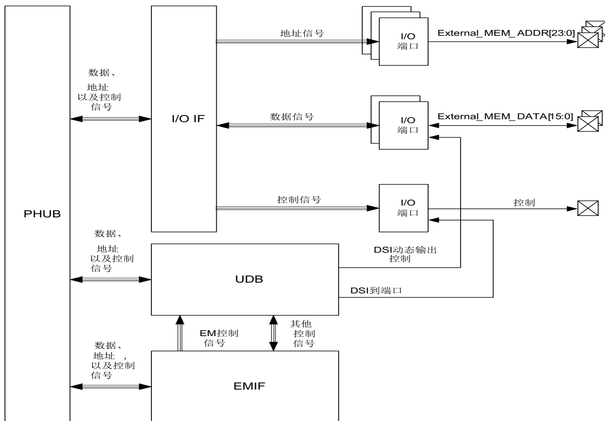
图 5-1. EMIF 框图
