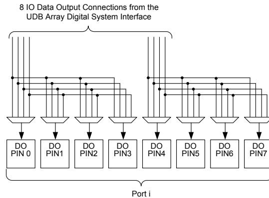
图 7-12. I/O 引脚输出连接
