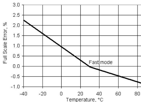
图 11-33. IDAC 全量程误差与温度，范围 = 255 \mu A，灌电流模式
