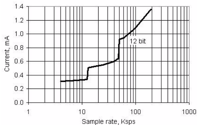
图 11-25. Delta-sigma ADC IDD 与 sps, 范围 = \pm 1.024 V, 连续采样模式, 旁路输入缓冲区
