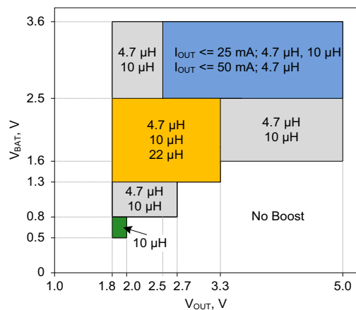
图 11-10. 在 V_{\text{BAT}} 与 V_{\text{OUT}} 范围内的 L_{\text{BOOST}} 值
