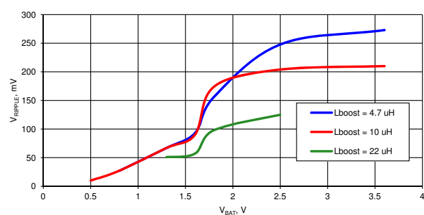
图 11-14. V_{RIPPLE} 与 V_{BAT} [34]
