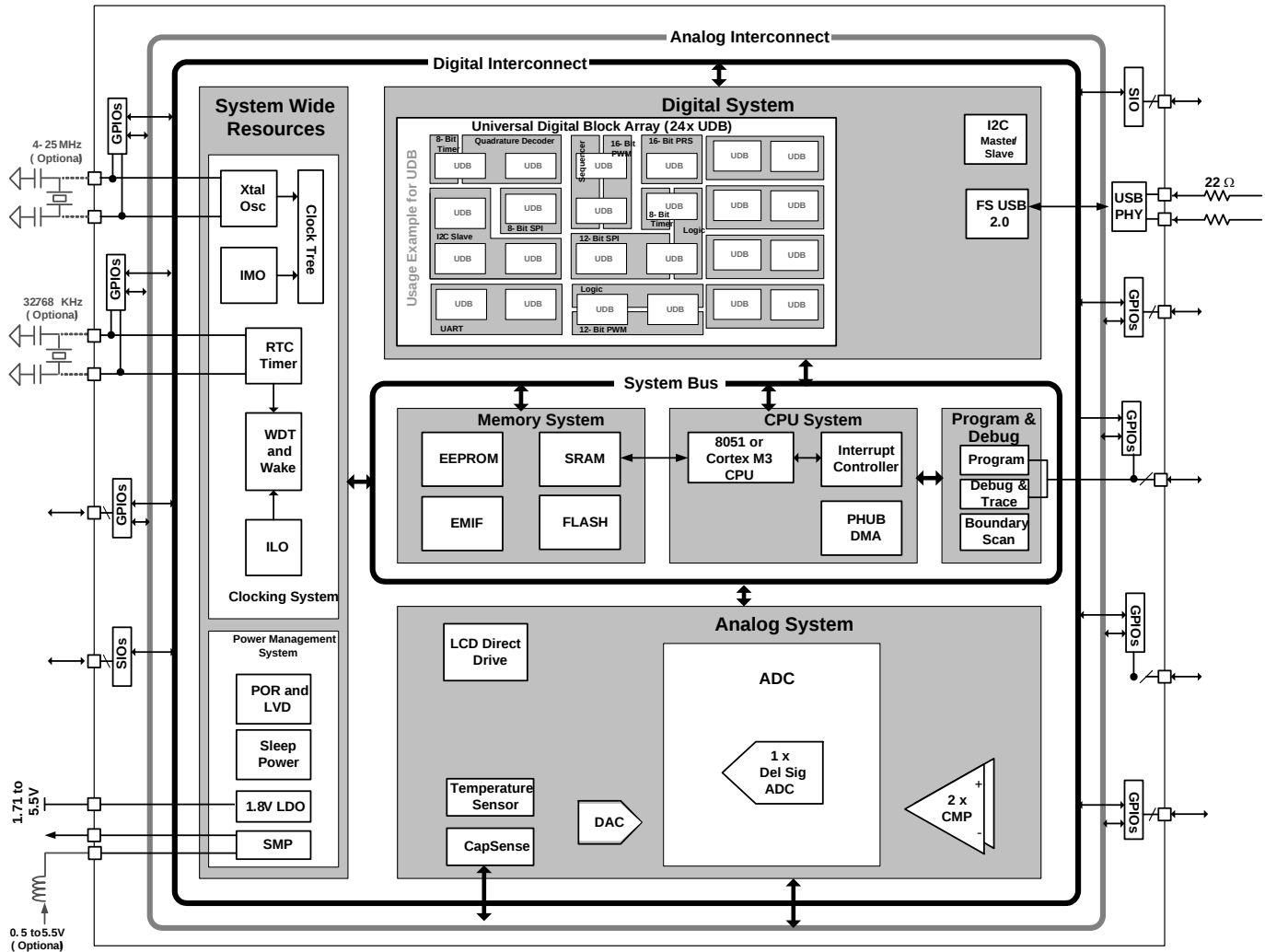
图 1-1. 简化的框图
