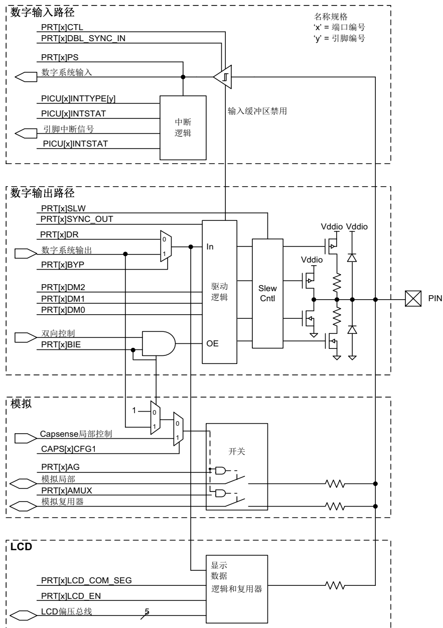
图 6-9. GPIO 框图
