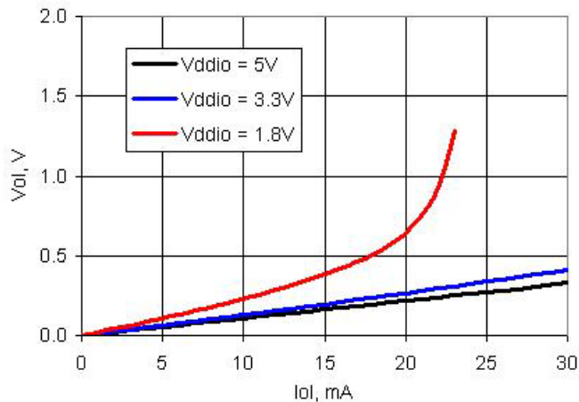
图 11-18. SIO 输出低电平和电流，非稳压模式
