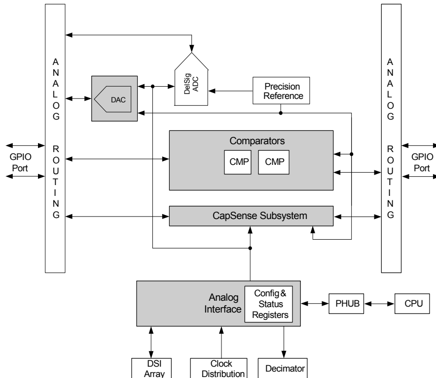
图 8-1. 模拟子系统框图
