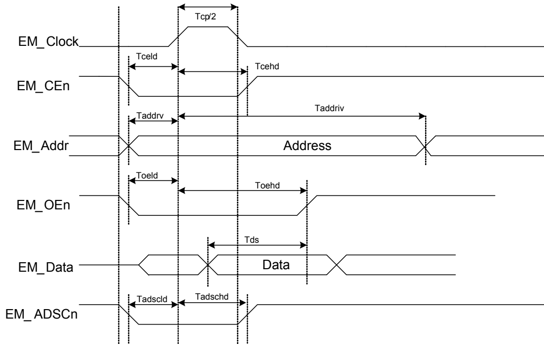
图 11-55. 同步读周期时序
