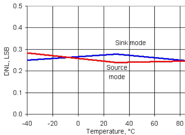
图 11-31. IDAC DNL 与温度，范围 = 255 \mu A，高速模式
