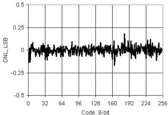
图 11-28. IDAC DNL 与输入代码，范围 = 255 \mu A，拉电流模式
