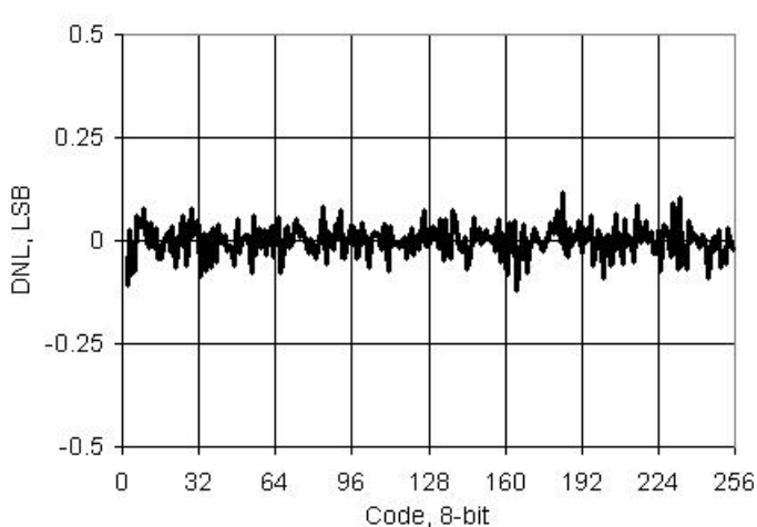
图 11-41. VDAC DNL 与输入代码，1 V 模式
