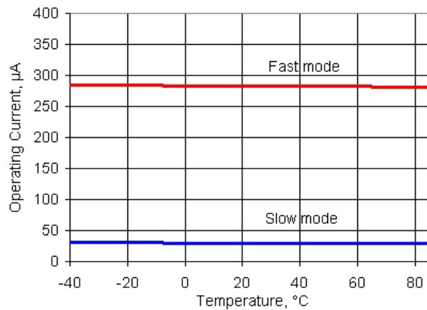
图 11-35. IDAC 工作电流与温度，范围 = 255 \mu A，代码 = 0，灌电流模式
