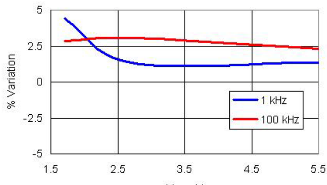
图 11-63. ILO 频率变化与 V_{DD}
