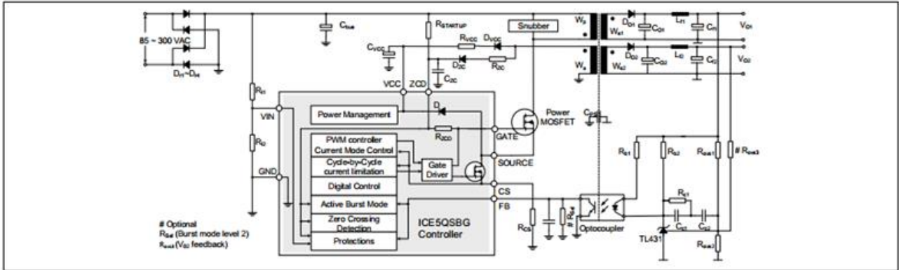
图 1 典型应用 表 1 第五代准谐振控制器的输出功率
