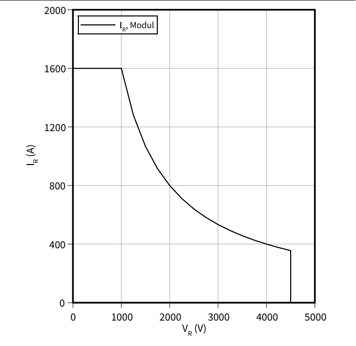
安全工作区 (SOA), 二极管, 逆变器 I_R = f(V_R) T_{vj} = 125\text{ °C}
