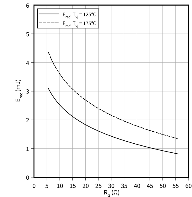
开关损耗（典型），二极管，逆变器 E_{rec} = f(R_G) I_F = 75 A , V_R = 600 V
