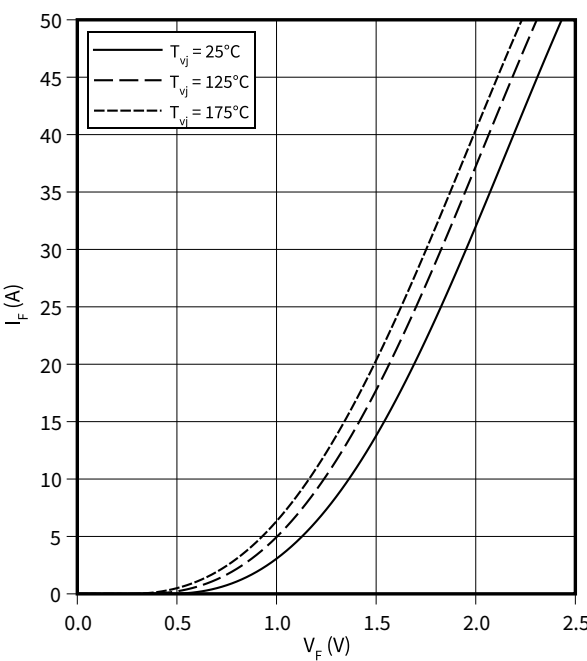
正向特性（典型），Diode-斩波器 I_F = f(V_F)
