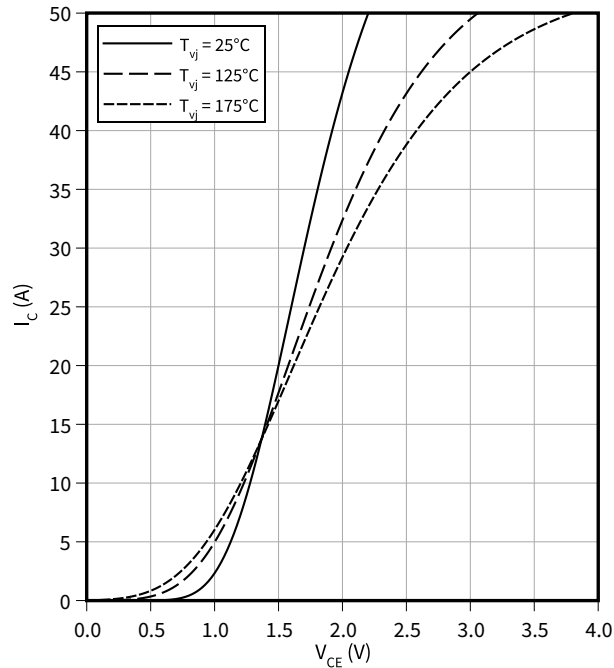
输出特性（典型），IGBT，斩波器 I_C = f(V_{CE}) V_{GE} = 15\text{ V}
