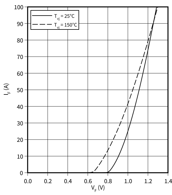
正向偏压特性 (典型), Diode-斩波器
