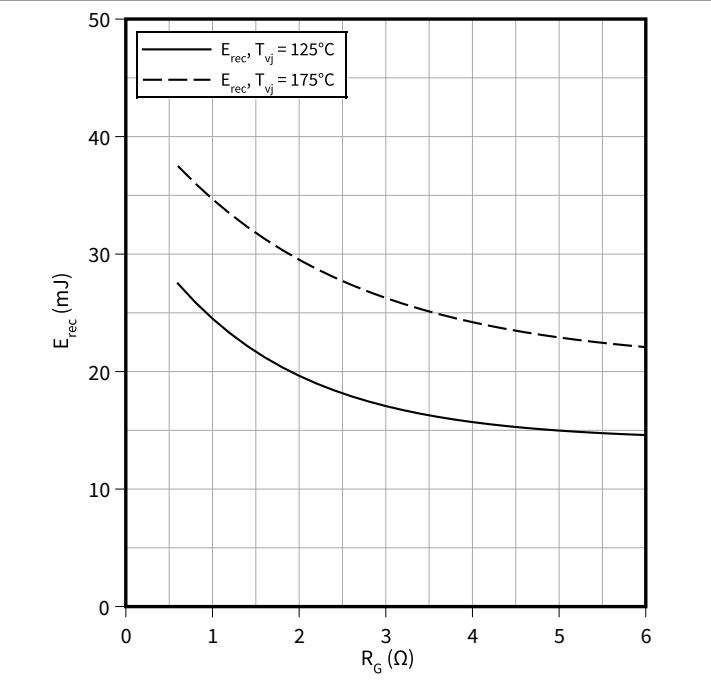
スイッチング損失 (typical), Diode、インバータ E_{rec} = f(R_G) I_F = 450 \text{ A} , V_{CC} = 600 \text{ V}
