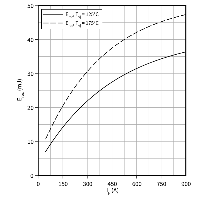
スイッチング損失 (typical), Diode、インバータ E_{rec} = f(I_F) R_{Gon} = 0.6 \Omega , V_{CC} = 600 \text{ V}
