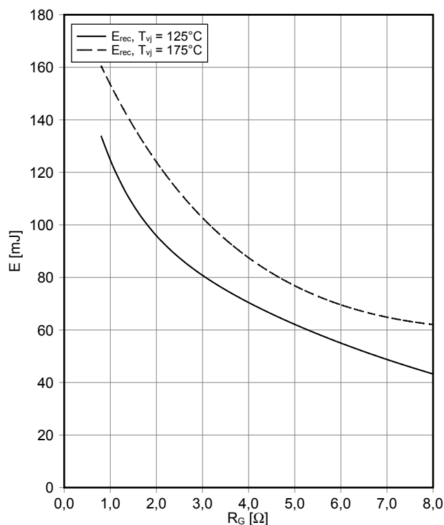
スイッチング損失 Diode、インバータ (Typical) switching losses Diode, Inverter (typical) E_{rec} = f(R_G) I_F = 1500 \text{ A} , V_{CE} = 600 \text{ V}
