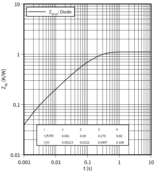
瞬态热阻抗 , 二极管, 整流器
