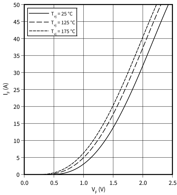
正向偏压特性 (典型), Diode-斩波器
