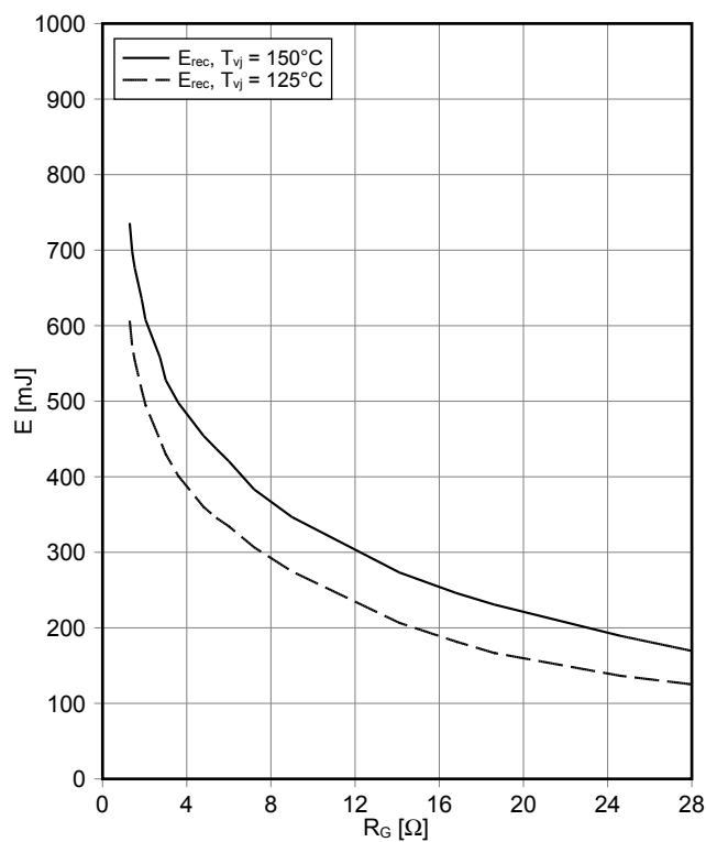
スイッチング損失 Diode、インバータ (Typical) switching losses Diode, Inverter (typical) E_{rec} = f(R_G) I_F = 500\text{ A} , V_{CE} = 1800\text{ V}
