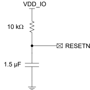
图 15. 复位连接
