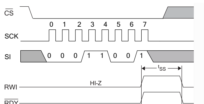
图 110. 自动存储禁用周期
