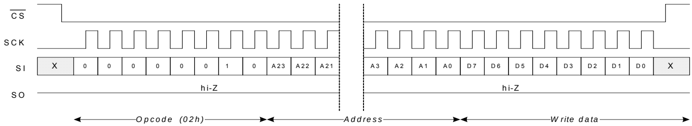
图 31. SPI 模式下的突发写指令
