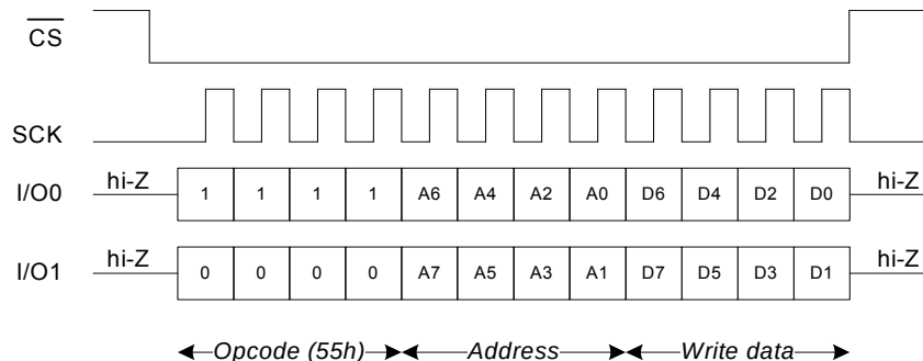
图 51. DPI 模式下的 WRRTC 指令
