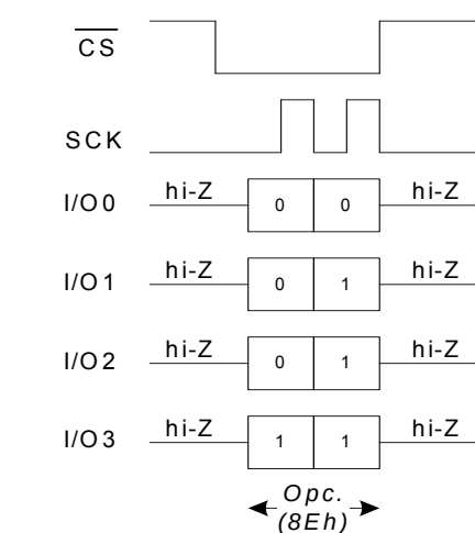
图 96. QPI 模式下的 ASEN 指令
