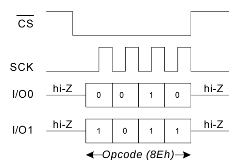
图 95. DPI 模式下的 ASEN 指令
