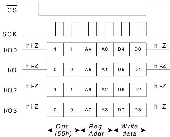
图 52. QPI 模式下的 WRRTC 指令
