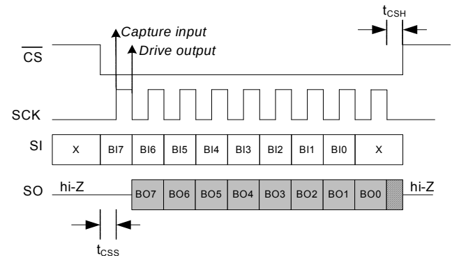
图 4. SPI 模式 0
