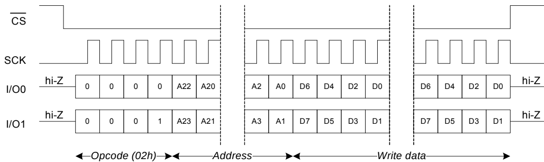
图 32. DPI 模式下的写指令
