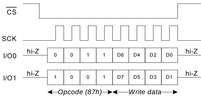
图 72. DPI 模式下的 WRCR 指令
