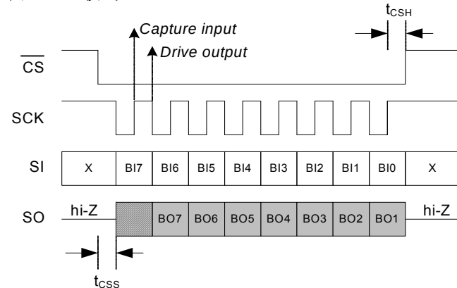
图 5. SPI 模式 3
