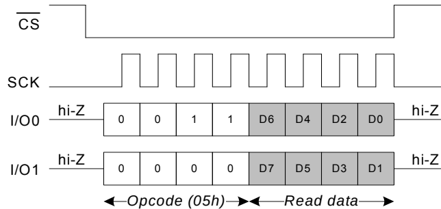
图 63. DPI 模式下的 RDSR 指令
