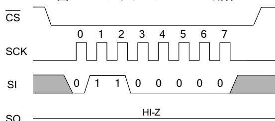
図 15. ソフトウェア RECALL 動作
