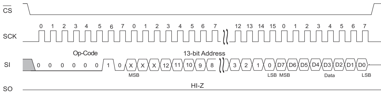
図 12. 書き込み命令タイミング
