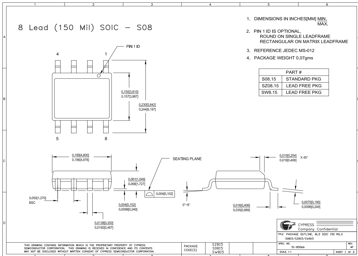
図 31. 8 ピン SOIC(150 ミル) パッケージの外形図、51-85066
