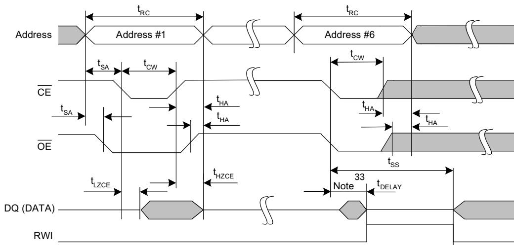
图 10. 自动存储使能 / 禁用周期 [32]
