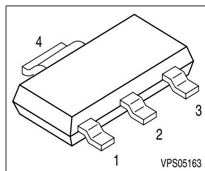
PG-SOT-223
