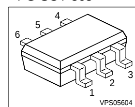
PG-SOT-363
