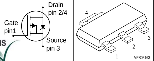
PG-SOT223
