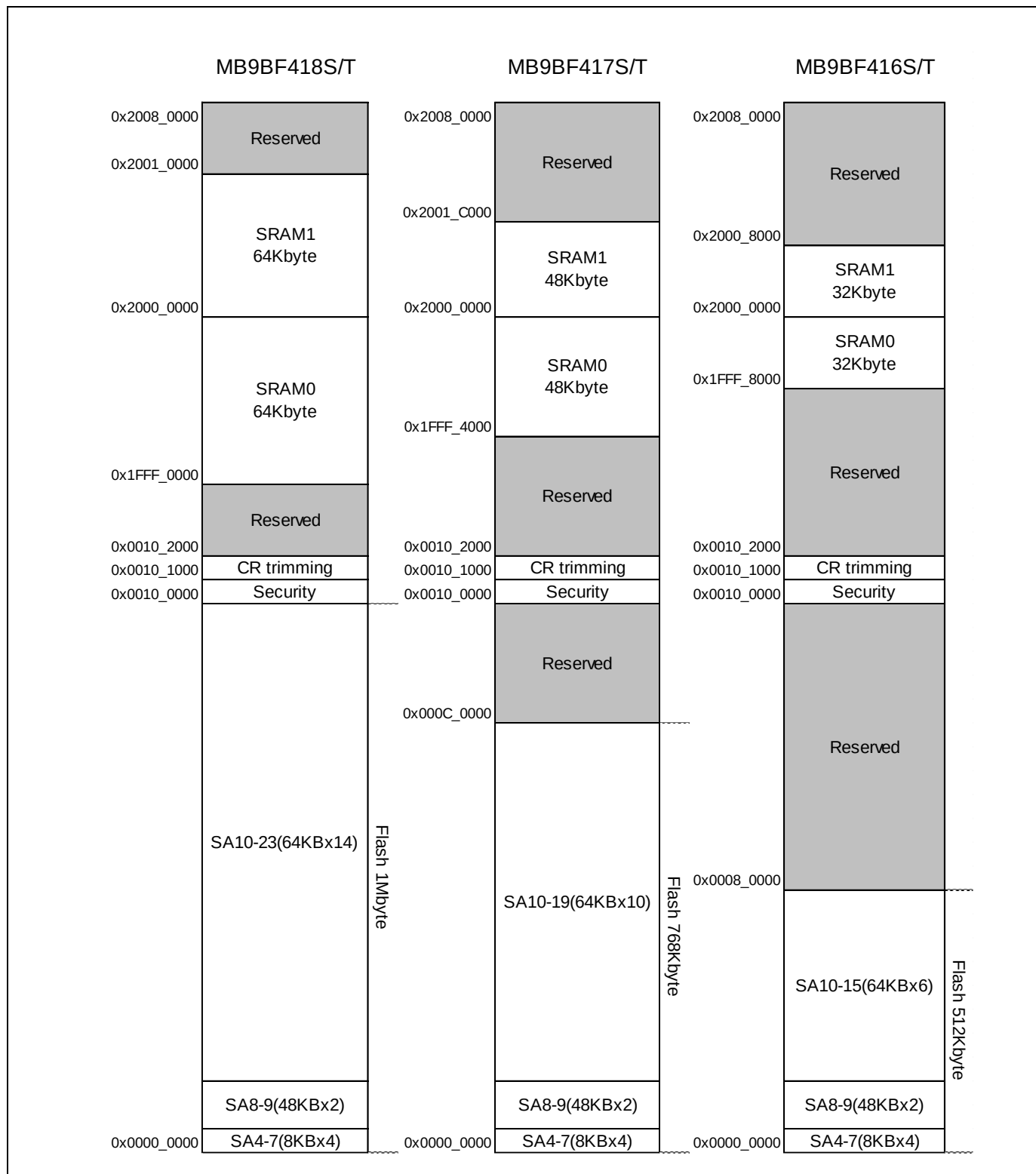
•Memory Map(2)
