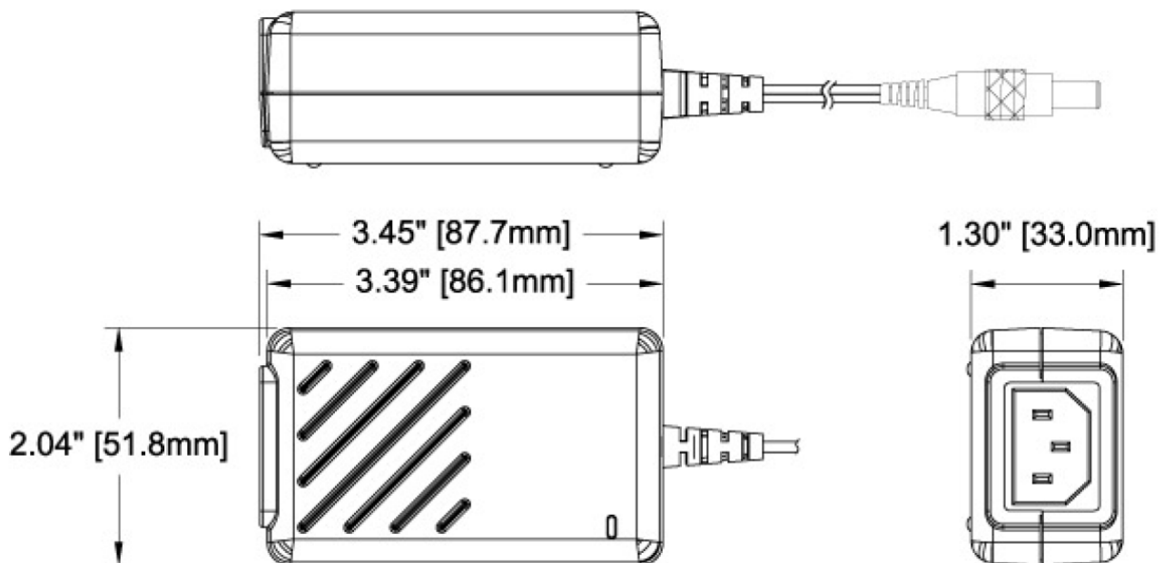
MWA020-DWG
