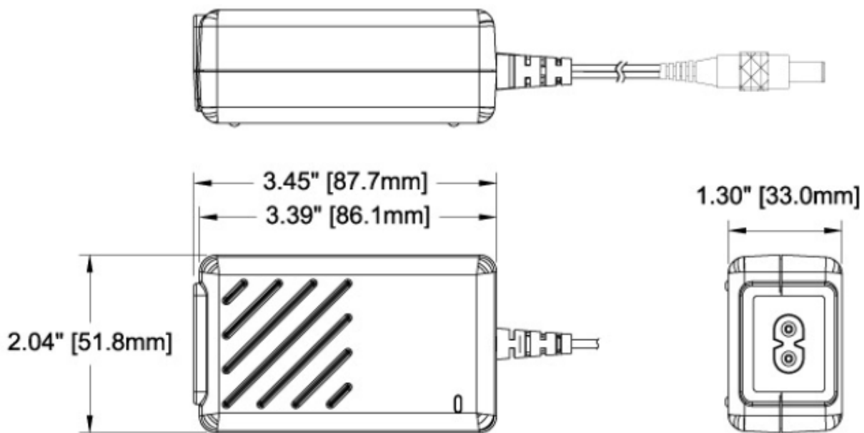
MWA020-DWG
