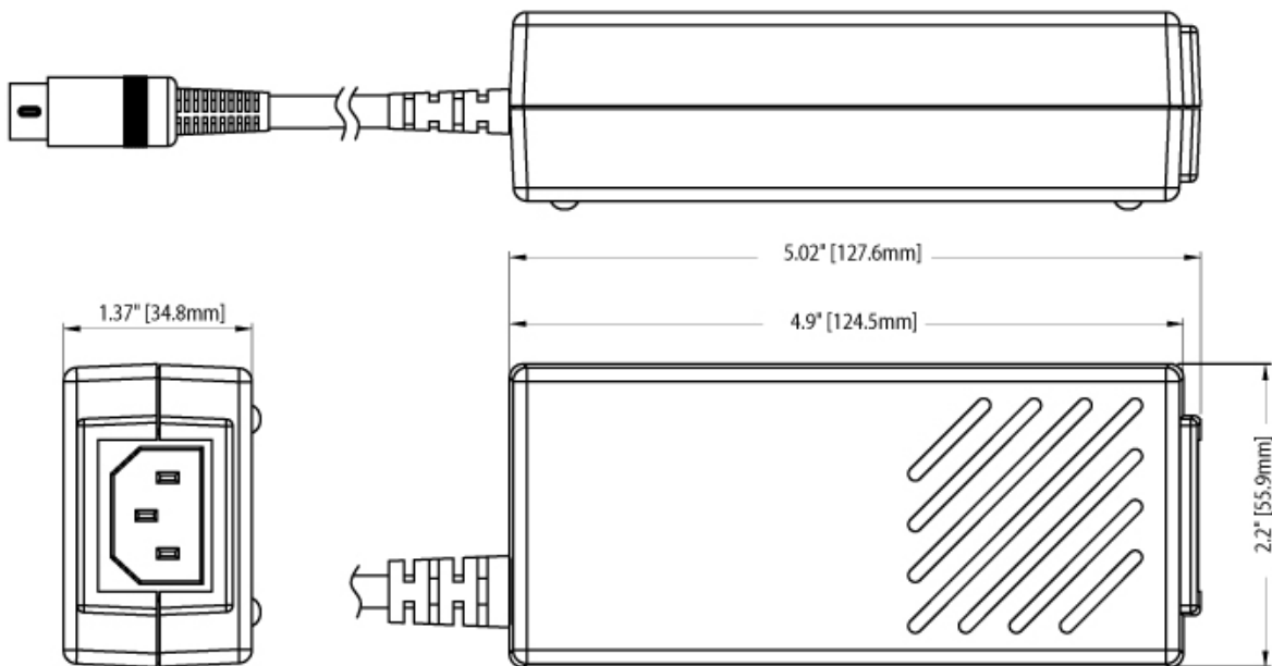
MWA065-Class I-DWG
