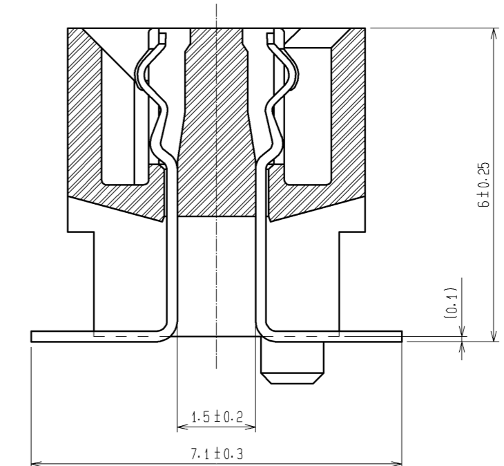
A-A (10:1)
