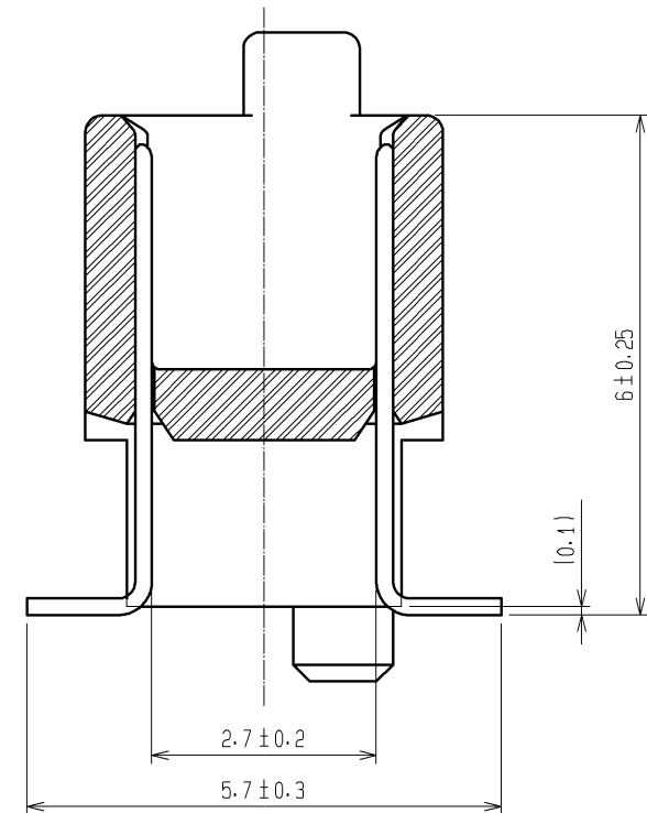
A-A (10:1)
