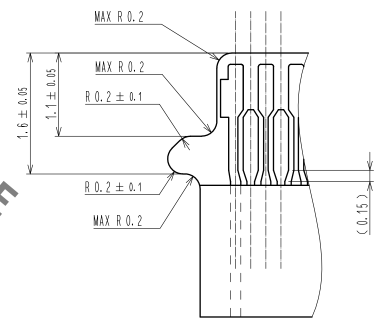
U (20 : 1)
