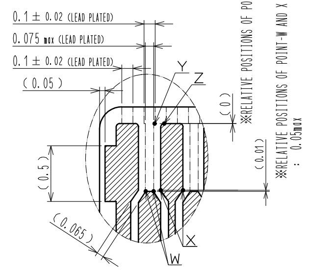
T (30 : 1)
