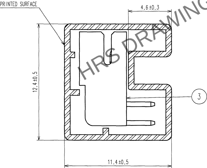
A-A (5:1)
