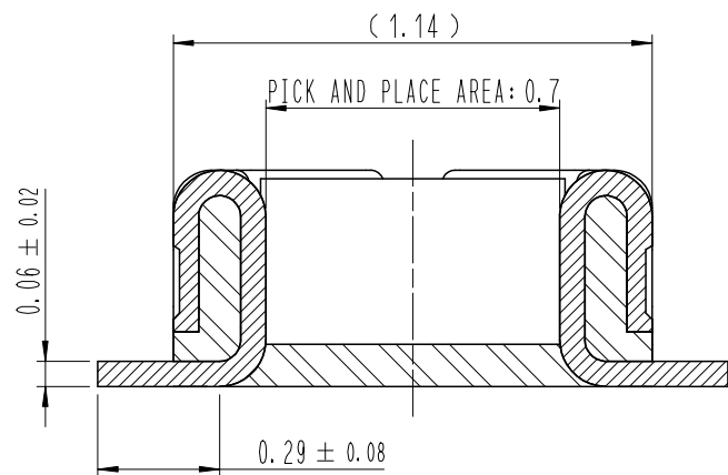
A-A (50:1)
