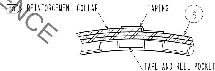
D-D (FREE)
