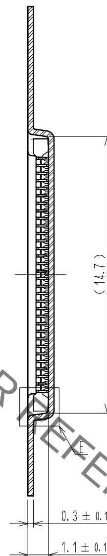
B-B (5:1)
