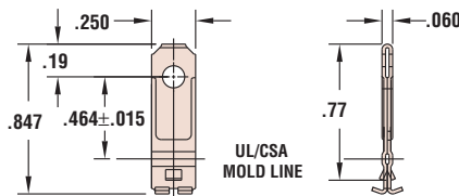
PCB 5201 2
