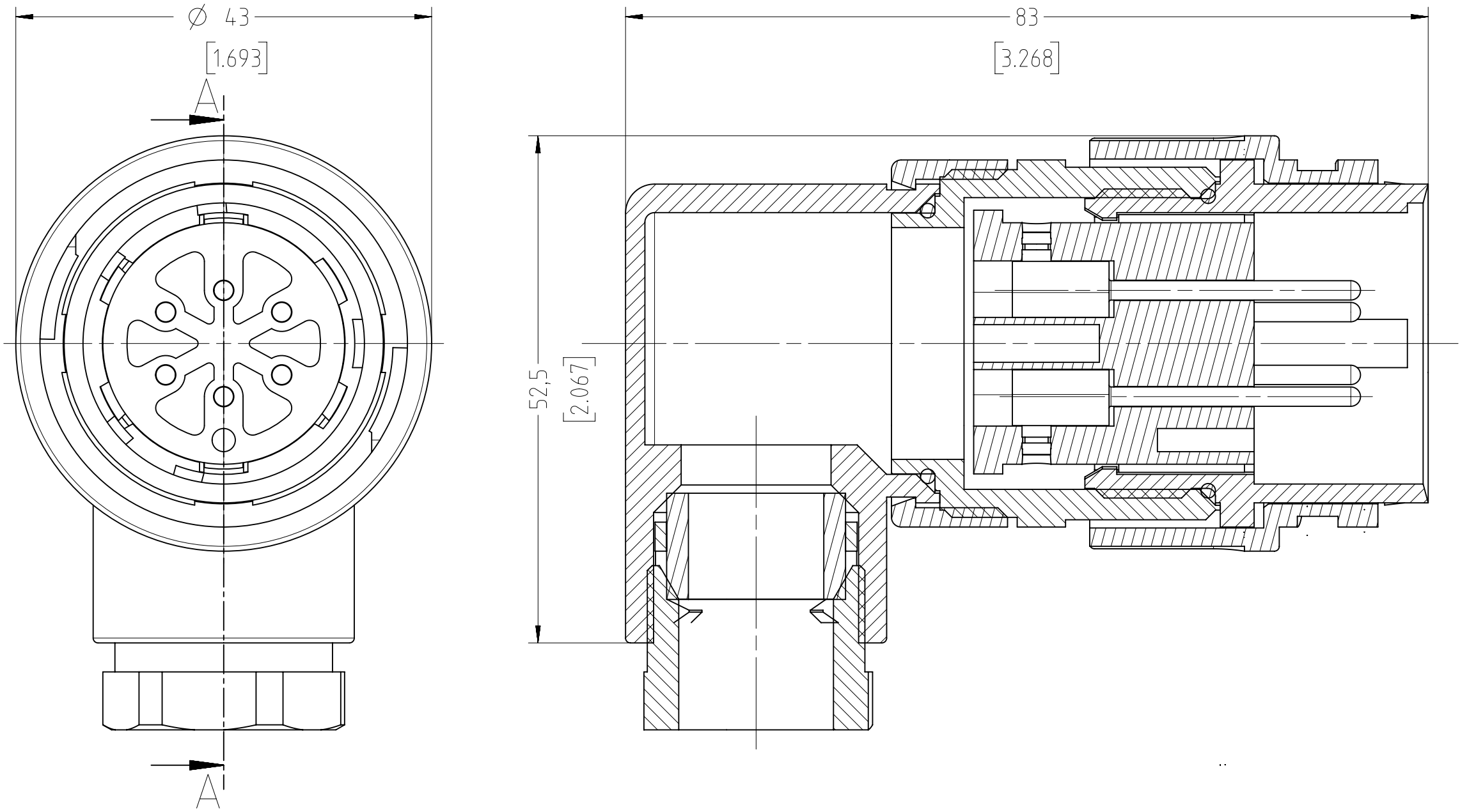
SCHNITT / SECTION A-A
