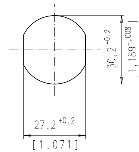
Montageausschnitt Panel cutout
