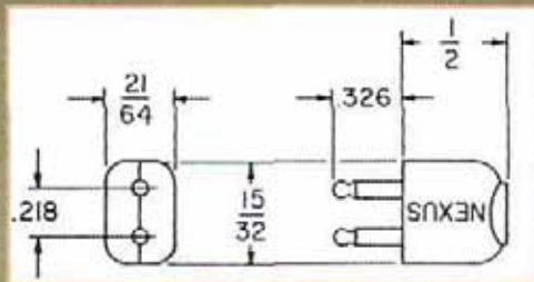
MP-101 (U-173/U)
