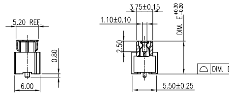
A-A SECTION
