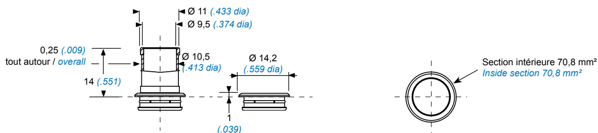
Cheminée cylindrique / Cylindrical chimney
