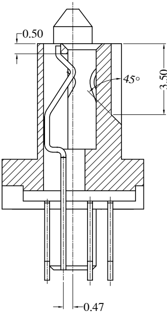
SECTION D-D
