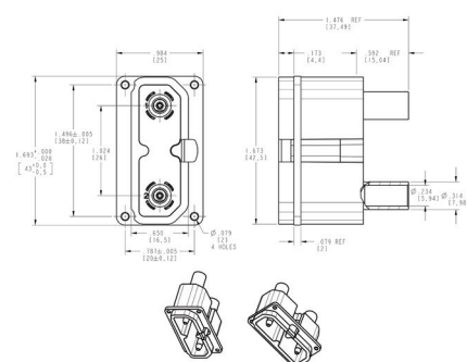
C10-752161-000 RADSOK® Receptacle, 1500V
