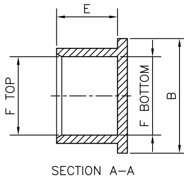
Dimension Table (Receptacle)
